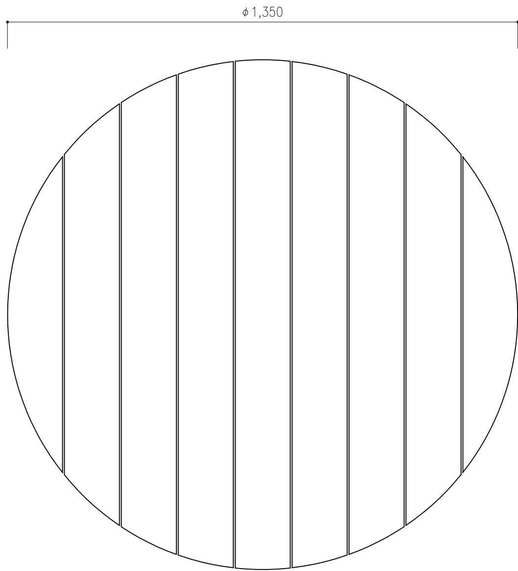
平面図
