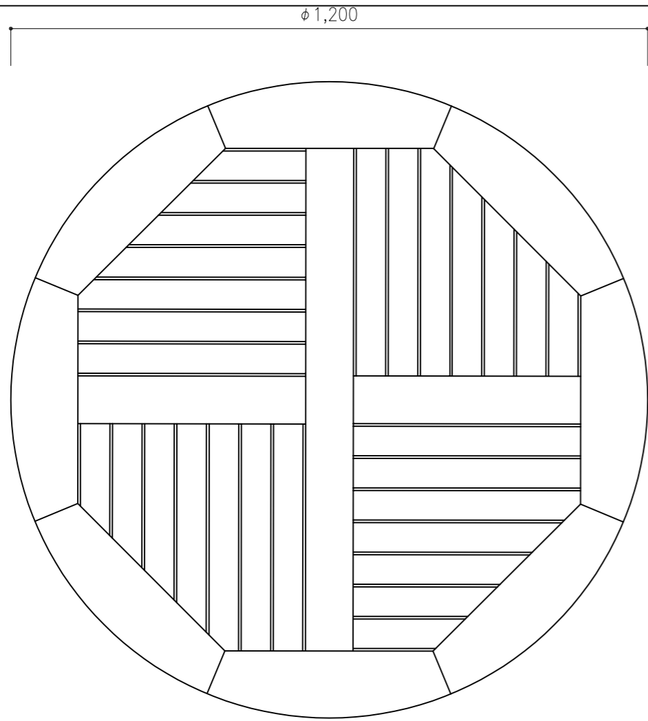
平面図
