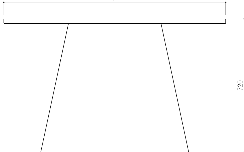
正面図
