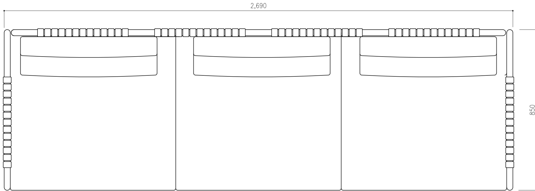
平面図
