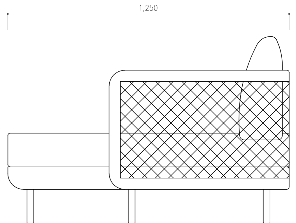
側面図
