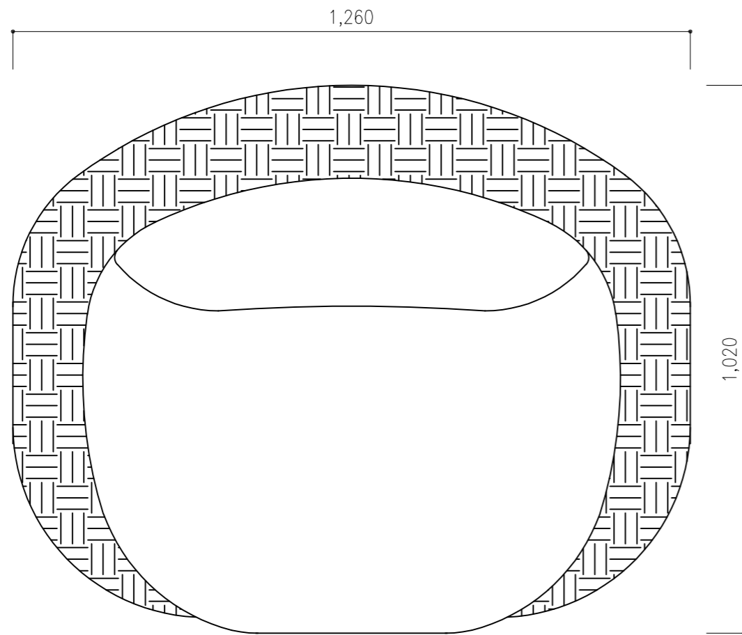
平面図
