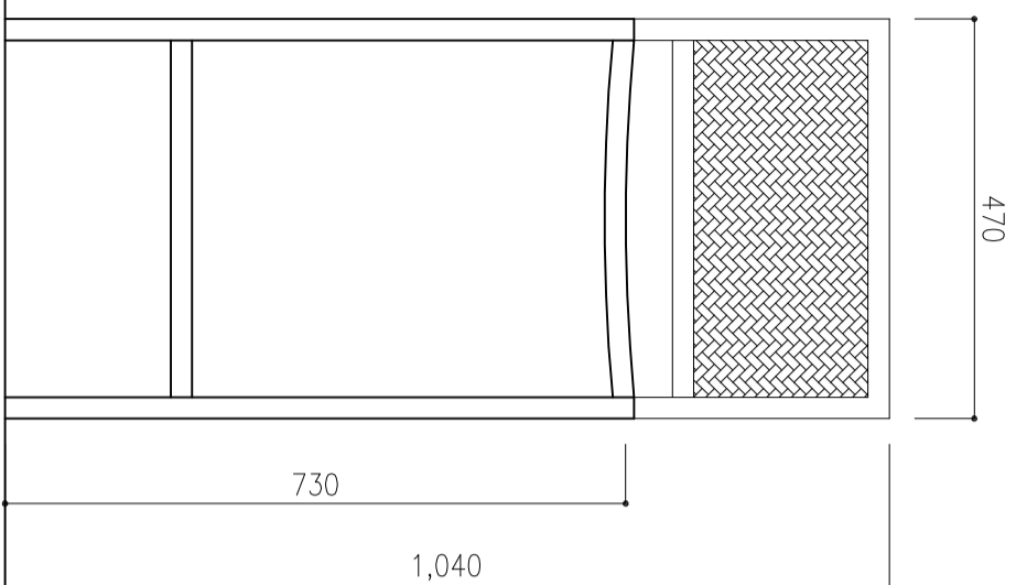
正面図
