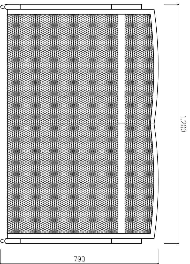
平面図
