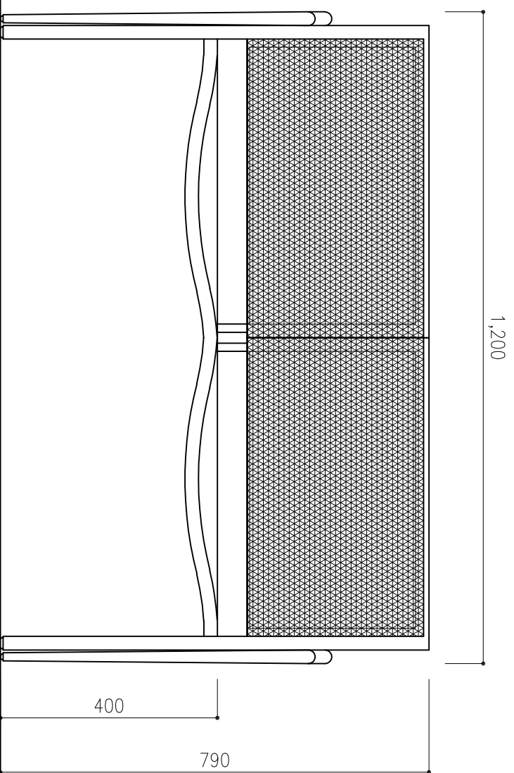
正面図
