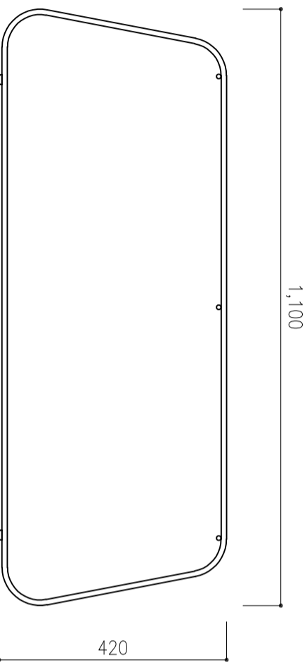
正面図
