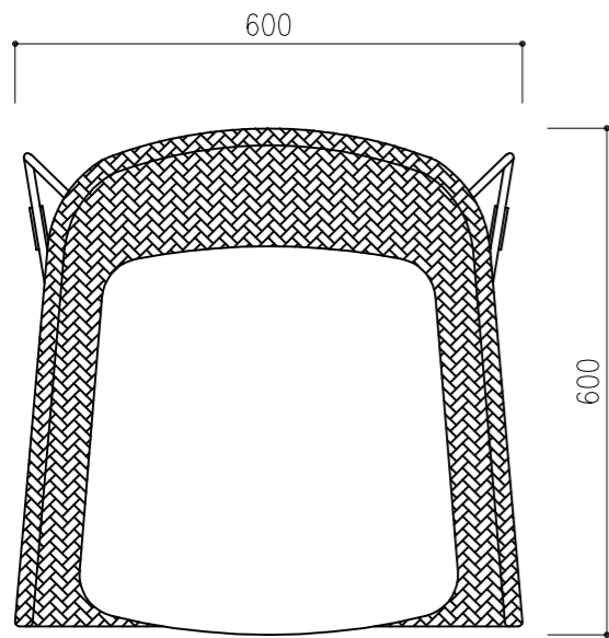
平面図
